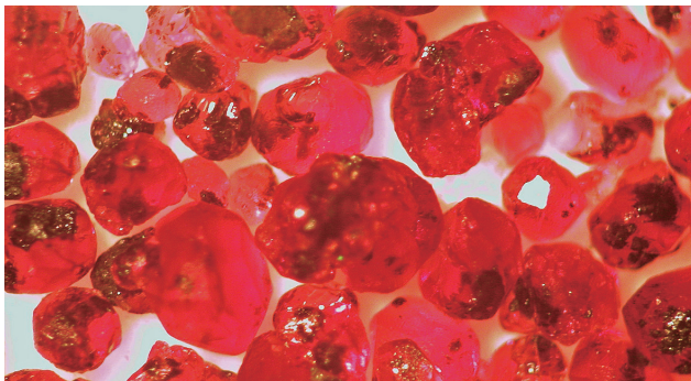
▲丹沢の衝突に伴う火山噴出物中のザクロ石
