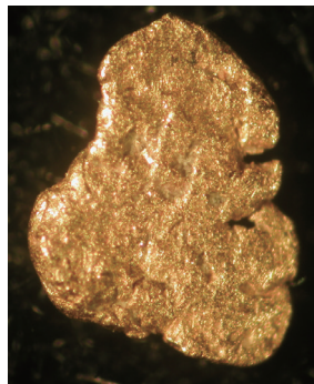
▲丹沢山地由来の砂金
