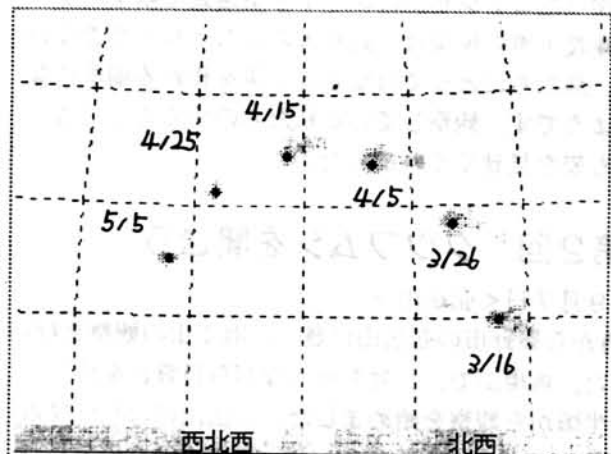
日没1時間後の彗星の位置（点線は10度おき）
